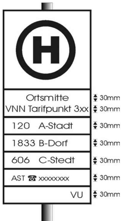
Abbildung 1: Haltestellenschild [eigene Zeichnung] der Kategorien 2 und 3
