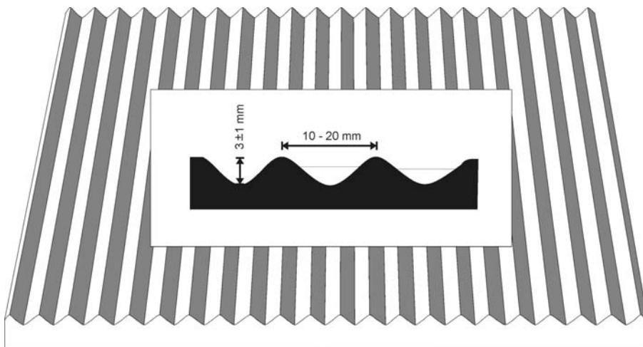
Abbildung 4: Rillenplatte als Oberflächengestaltung tastbarer Leistestreifen [eigene Zeichnung]
