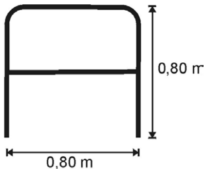
Abbildung 6: Rahmenhalter für Fahrräder [eigene Zeichnung nach ERA 95]
