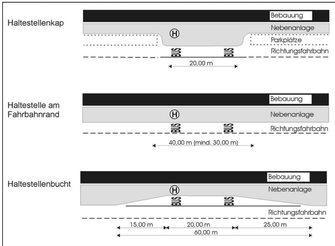
Abbildung 5: Haltestellentypen im Vergleich [eigene Zeichnung]
